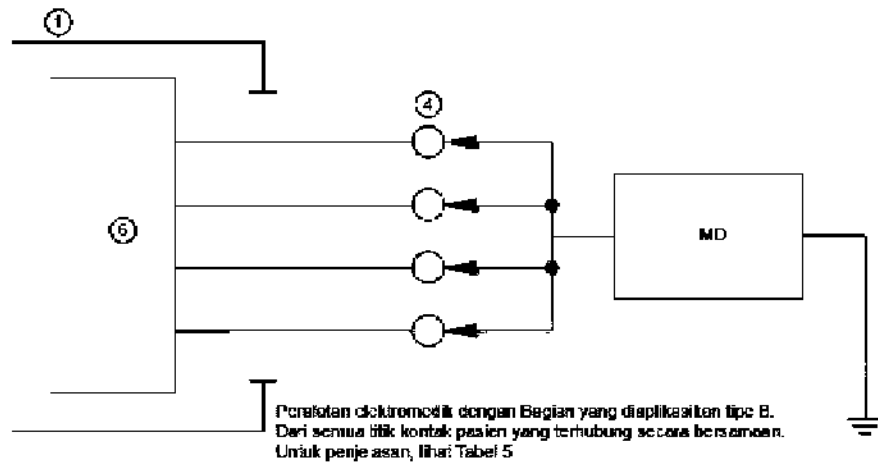
Gambar E.1 – Bagian yang diaplikasikan tipe B
