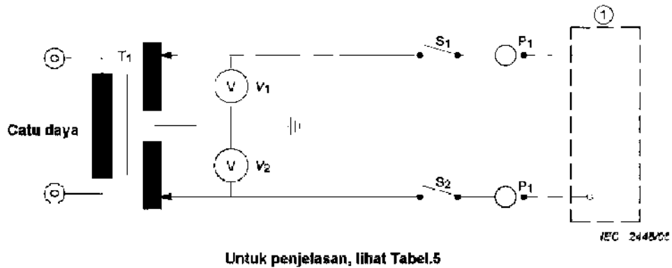
Gambar F.2 – Sirkuit catu daya pengukur dengan catu daya utama pada potensial pembumian simetris (lihat 8.7.4.2)
