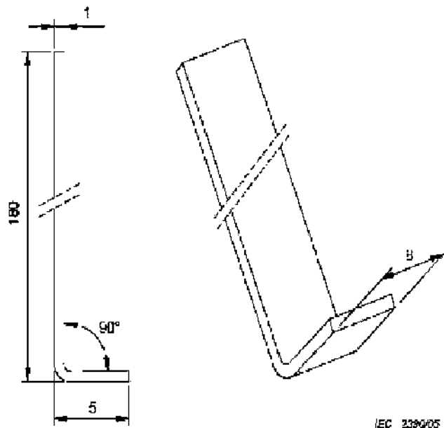
Gambar 7 – Kail uji (lihat 5.9.2.2)
