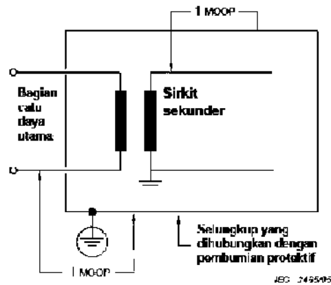
Gambar J.1 – Isolasi contoh 1
