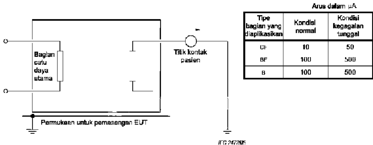
Contoh sirkuit pengukur catu dari Gambar F.1
