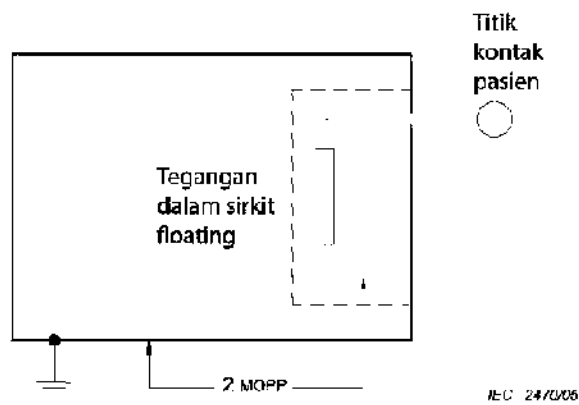
Gambar J.6 – Isolasi contoh 6
