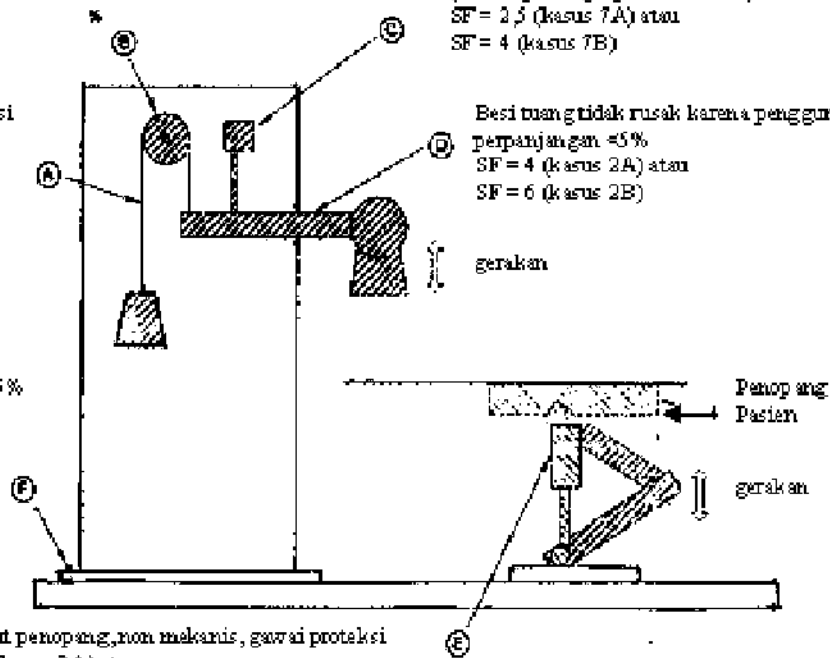
Gambar A.17 – Contoh dalam menentukan faktor keselamatan regangan menggunakan Tabel 21
