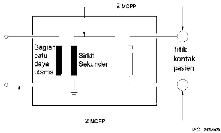
Gambar J.5 – Isolasi contoh 5
