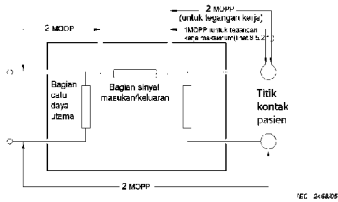
Gambar J.4 – Isolasi contoh 4
