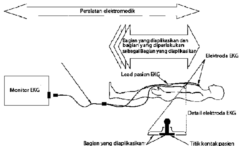
Gambar A.1 - Identifikasi peralatan elektromedik, bagian yang diaplikasikan dan titik kontak pasien pada monitor EKG
