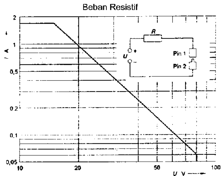
Gambar 35. Arus maksimum yang diizinkan/sebagai fungsi dari tegangan maksimum U yang terukur dalam suatu rangkaian resistif dalam lingkungan yang kaya oksigen (lihat 11.2.2.1)
