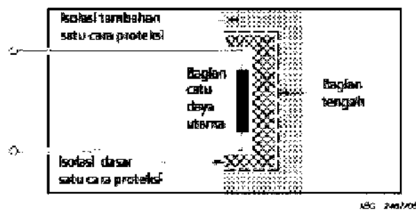
Gambar J.3 – Isolasi contoh 3
