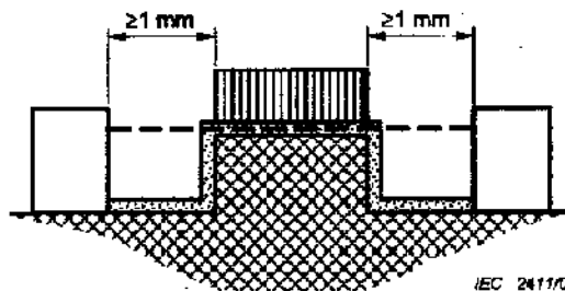
Gambar 28 - Jarak rambat dan celah udara – Contoh 7
