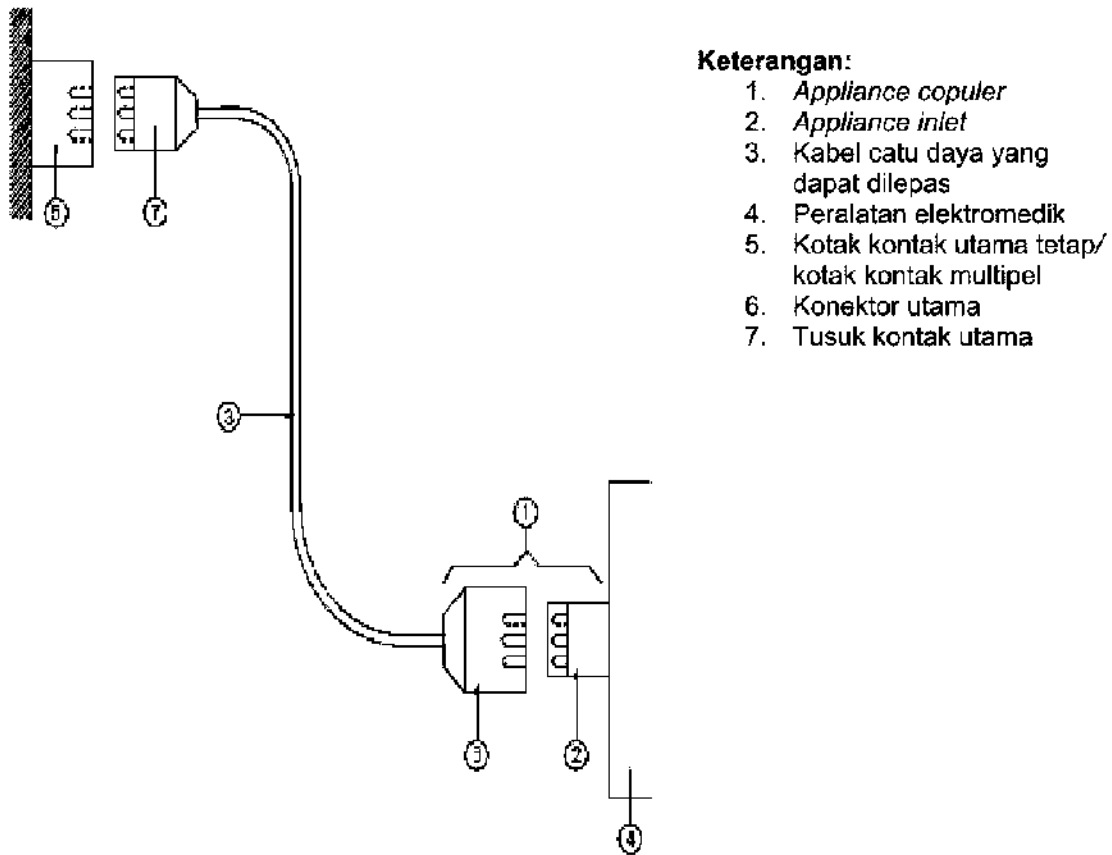
Gambar 1 – Sambungan utama yang dapat dilepas (lihat definisi)
