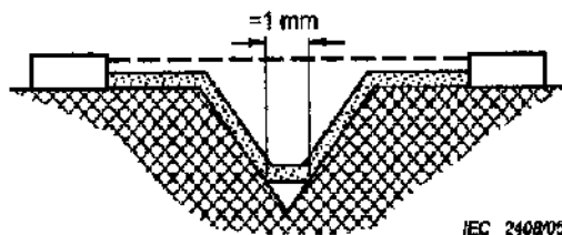
Gambar 24 - Jarak rambat dan celah udara – Contoh 3
