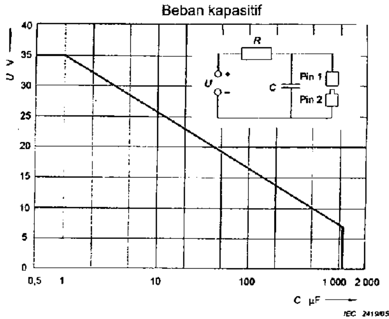
Gambar 36 – Tegangan maksimum U yang diizinkan sebagai fungsi dari digunakannya sirkuit kapasitansi C terukur dengan menggunakan sirkuit kapasitif lingkungan yang kaya oksigen (lihat 11.2.2.1)
