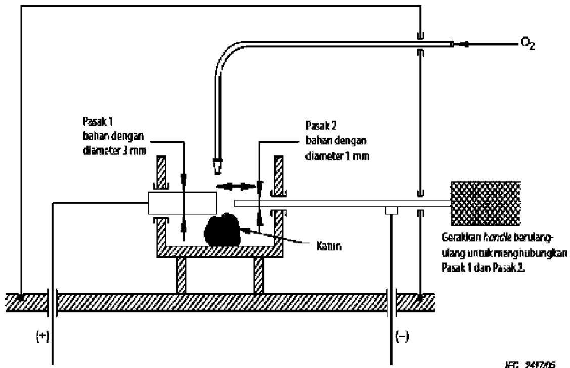
Gambar 34 – Alat uji percikan api penyalan (lihat 11.2.2.1)
