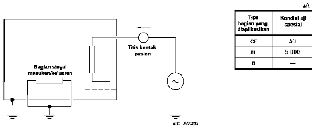
Contoh sirkuit pengukur catu dari Gambar F.1
