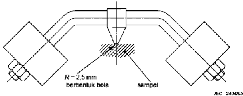
Gambar 21 – Alat pengujian tekanan bola (lihat 8.8.4.1)
