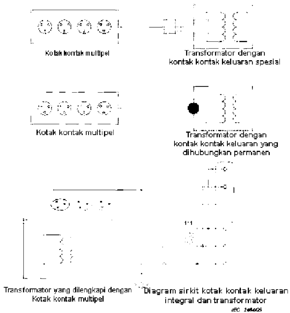
Gambar I.2 – Contoh aplikasi kotak kontak keluaran multipel
