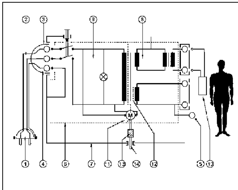
Gambar 3 – Contoh peralatan elektromedik kelas I (lihat definisi)
