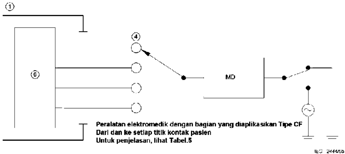
Gambar E.3 – Bagian yang diaplikasikan tipe CF
