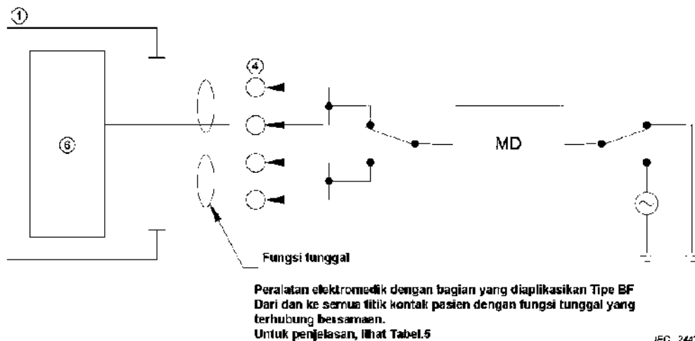
Gambar E.2 – Bagian yang diaplikasikan tipe BF
