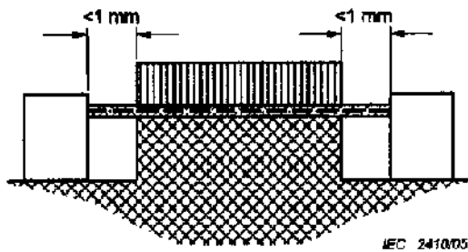
Gambar 27 - Jarak rambat dan celah udara – Contoh 6
