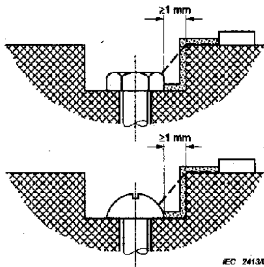
Gambar 29 - Jarak rambat dan celah udara – Contoh 8
