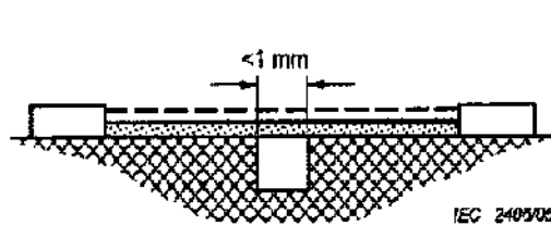
Gambar 22 - Jarak rambat dan celah udara – Contoh 1
