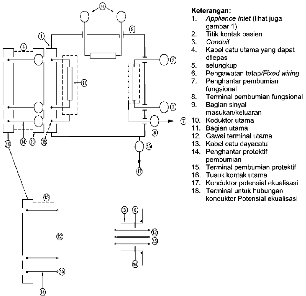
Gambar 2 – Contoh penghantar dan terminal (lihat definisi)
