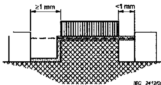
Gambar 29 - Jarak rambat dan celah udara – Contoh 8
