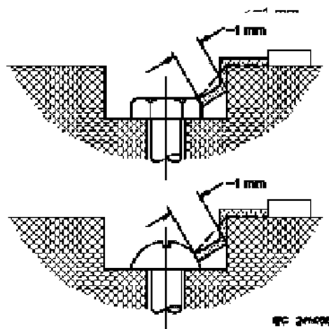
Gambar 31 - Jarak rambat dan celah udara – Contoh 10
