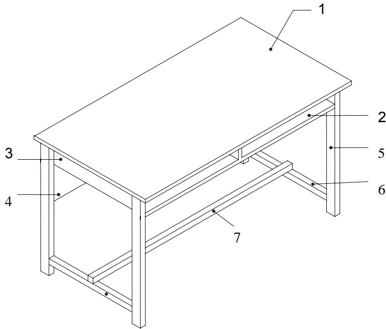
Gambar 1 – Bagian meja
