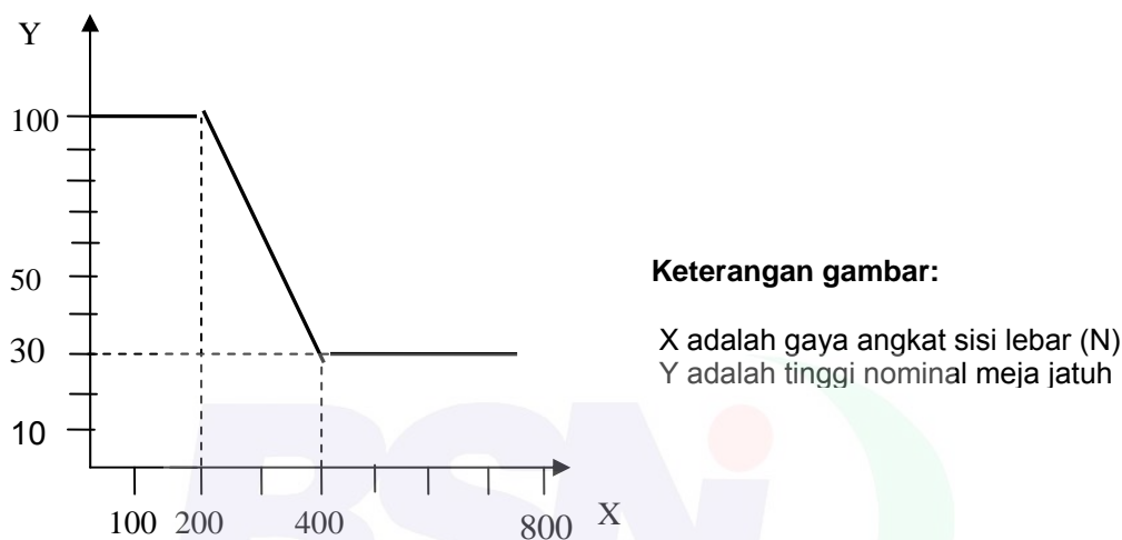
Gambar 11 – Grafik penentuan tinggi uji jatuh
