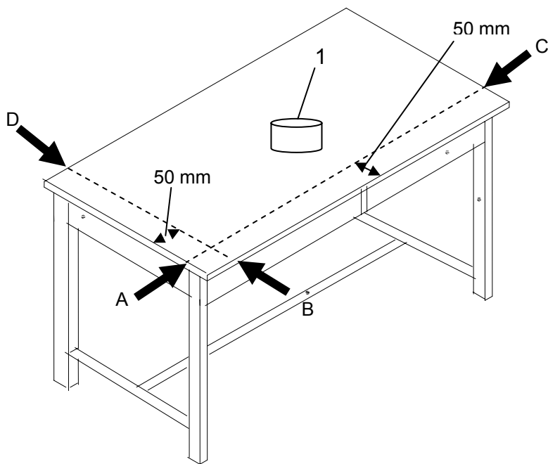
Gambar 7 – Uji ketahanan meja gaya horizontal
