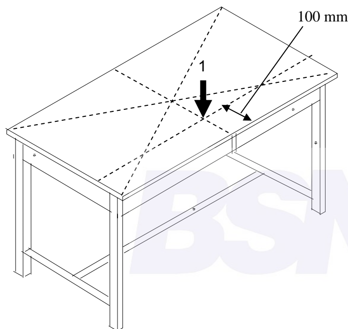
Gambar 3 – Uji stabilitas meja gaya vertikal
