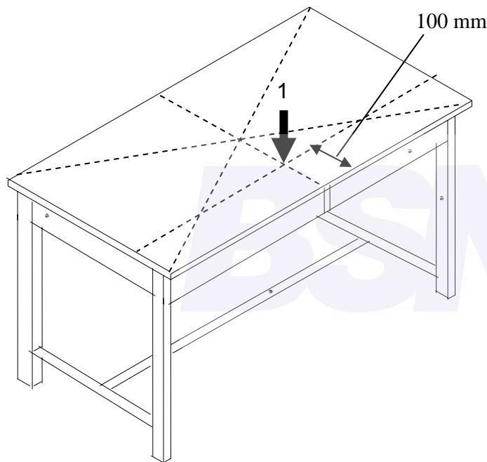
Gambar 6 – Uji ketahanan meja gaya vertikal
