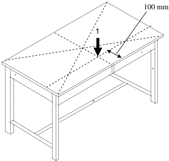
Gambar 4 – Uji kekuatan meja gaya vertikal
