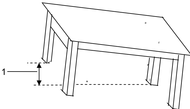
Gambar 10 – Uji jatuh meja
